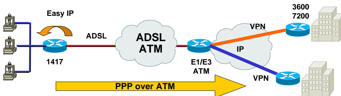
Fig. 3.12: VPN utilizzando Easy IP e ADSL (in architettura PPPoA)
